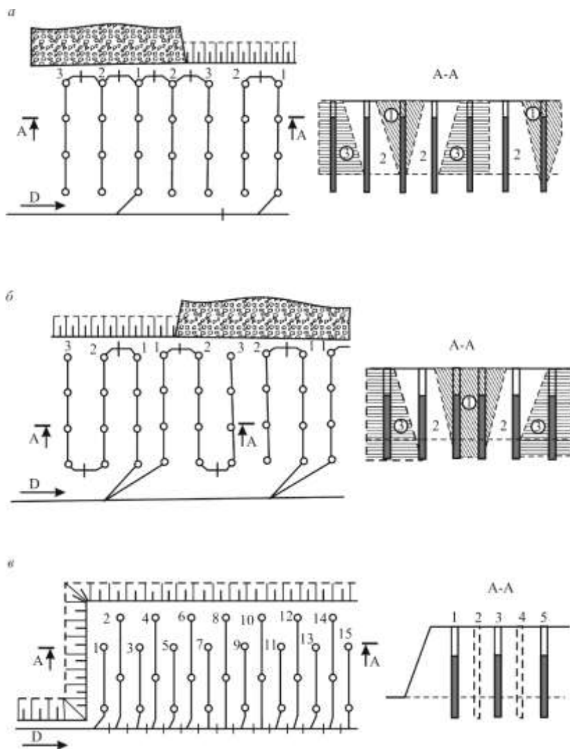
Рис. 6.10. Схеми з'єднання зарядів при поперечному підірванні рядів
