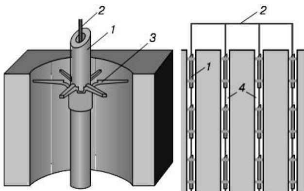
Рис. 7.29. Схема розташування еластичних трубочастих зарядів "Гранілен" в шпурах:
