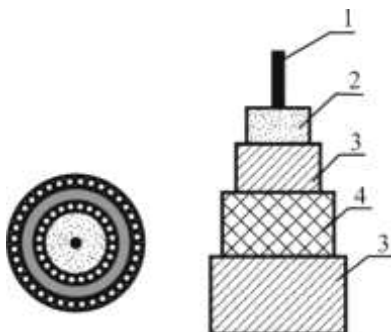
Рис. 3.2. Конструкція вогнепровідного шнура
