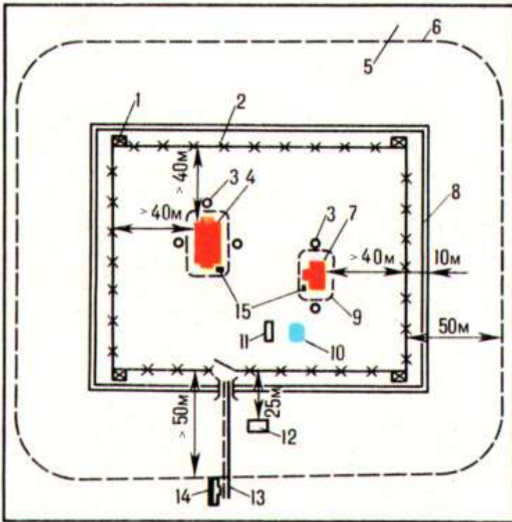
Рис. 8.1. Схема території складів ВМ
