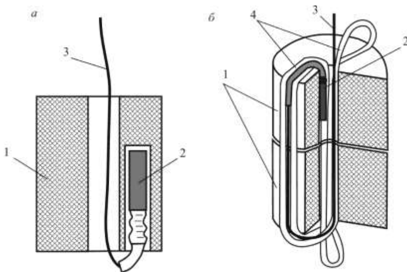
Рис. 4.31. Схема з'єднання пристрою УНС-С з шашкою Т- 400Г
