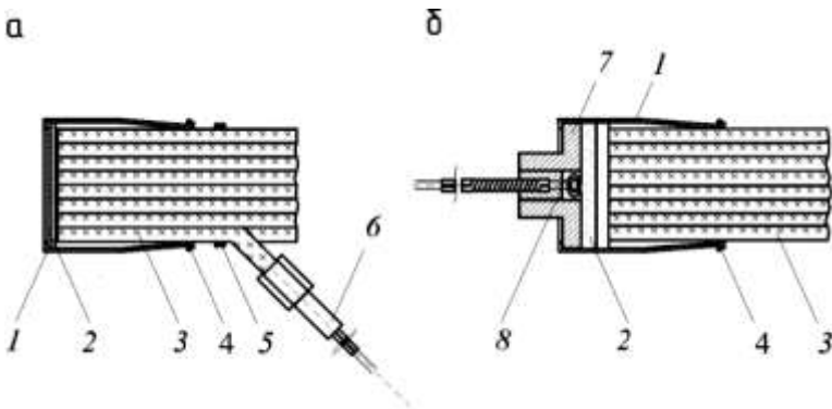
Рис. 3.5. Засоби запалювання ВШ: а – запалювальний патрон; б – електрозапалювальний патрон
