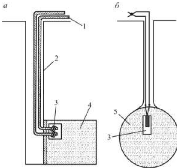
Рис. 5.4. Зосереджені заряди:
