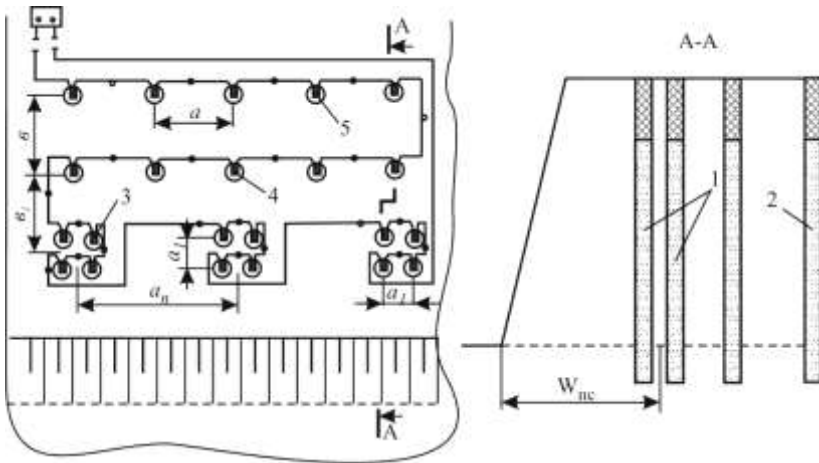
Рис. 7.23. Схема короткосповільненого підривання паралельно зближених зарядів:
