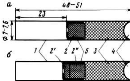
Рис. 3.1. Капсуль-детонатор:
