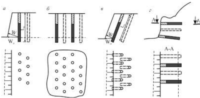
Рис. 7.2. Руйнування порід методом шпурових зарядів
