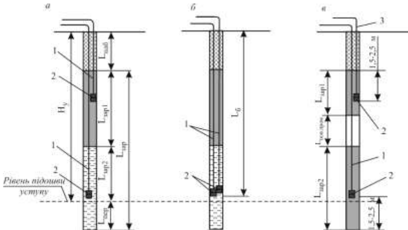
Рис. 4.38. Схема конструкції свердловинного заряду
