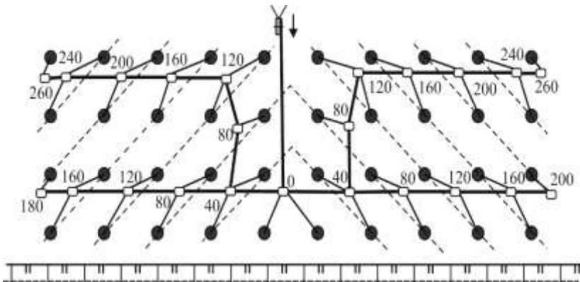
Рис. 4.36. Клинова монтажна схема ініціювання за допомогою УНС-ПА-40 або УНС-П-40
