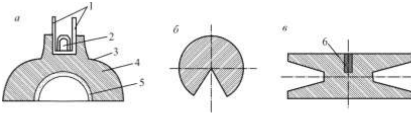
Рис. 7.16. Конструкція кумулятивних зарядів:
