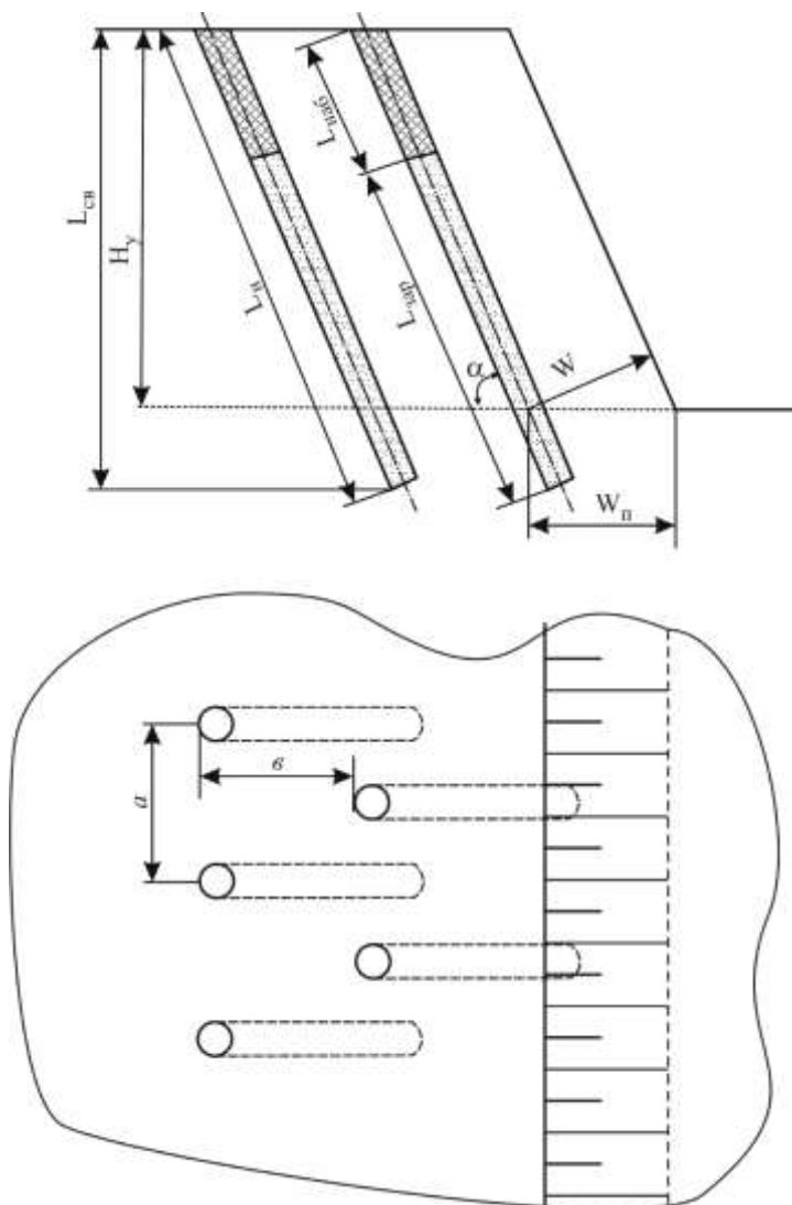
Рйис. 7.6. Схема розташування похилих свердловин
