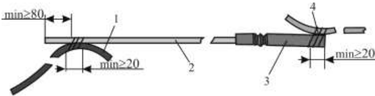
Рис. 4.30. Схема з'єднання хвилеводів з ДШ або ЕД.
