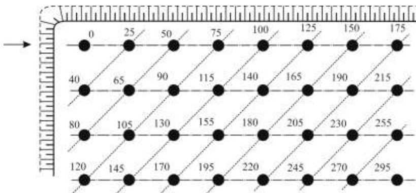
Рис. 4.33. Діагональна схема ініціювання зарядів ВР з використанням УНС-ПА-40 або УНС-П-40
