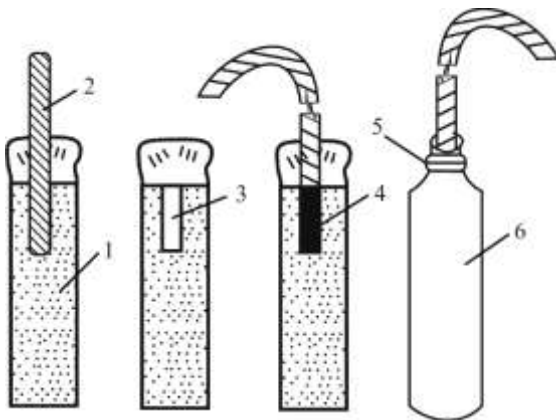
Рис. 4.1. Виготовлення бойовика при вогневому підірванні
