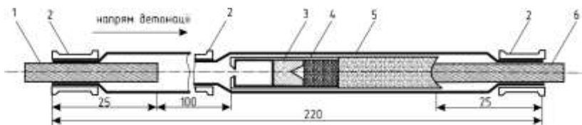
Рис. 3.10. Піротехнічний сповільнювач КЗДШ-69
