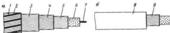
Рис. 3.8. Конструкція ДШ
