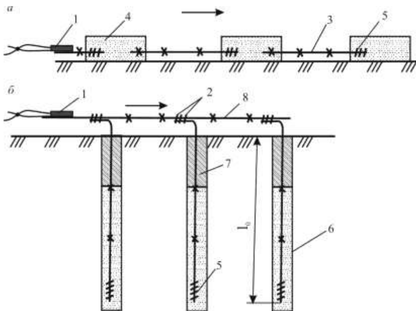
Рис. 4.20. Схеми вибухових мереж з ДШ:
