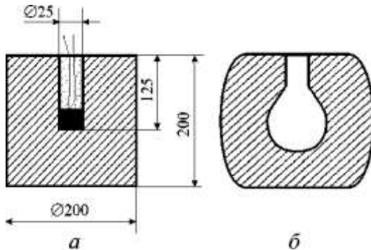
Рис. 1.2. Схема визначення працездатності ВР в свинцевій бомбі:
