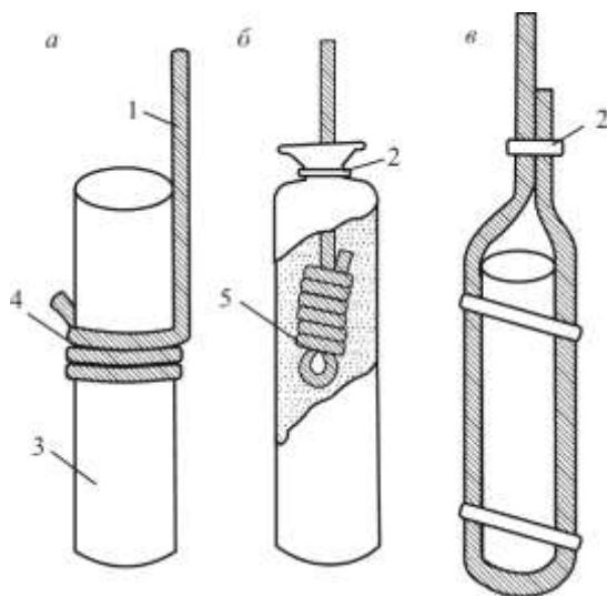
Рис. 4.22. Конструкція бойовиків при підриванні детонуючим шнуром:
