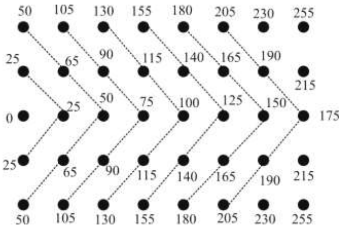
Рис. 4.34. Клинова схема ініціювання з використанням пристроїв УНС-ПА-25 або УНС-П-25
