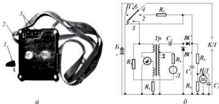
Рис. 4.4. Конденсаторний підливний прилад КВП-1/100м:
