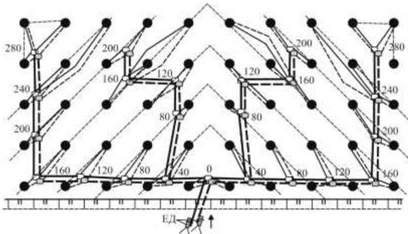
Рис. 4.34. Клинова схема ініціювання з використанням пристроїв УНС-ПА-25 або УНС-П-25
