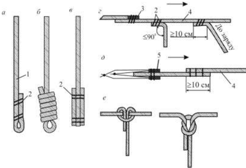
Рис. 4.19. Конструкція детонаційних вузлів ДШ і способи його з'єднання: 1 – відрізок ДШ; 2 – шпигат; 3 – запалювальна трубка; 4 – магістраль ДШ
