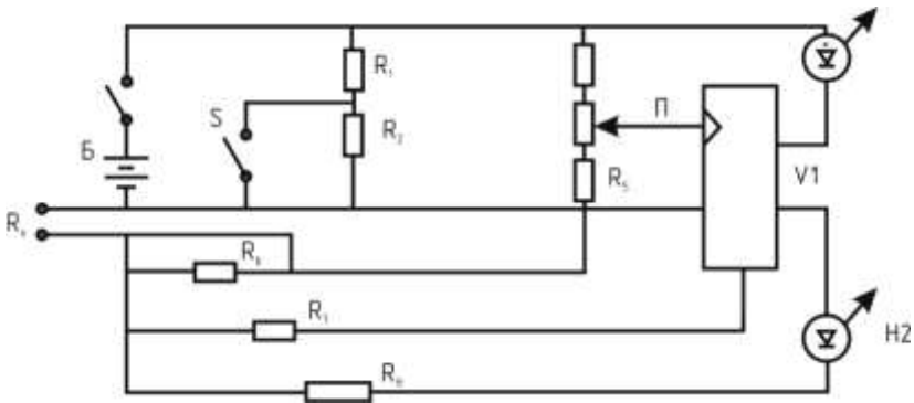
Рис. 4.9. Електрична схема мосту P-3043
