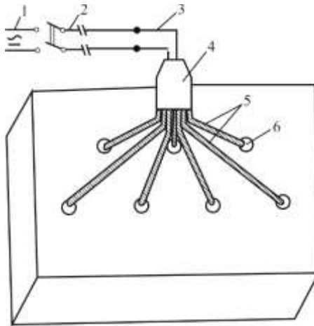
Рис. 4.18. Схема електровогневого підривання:
