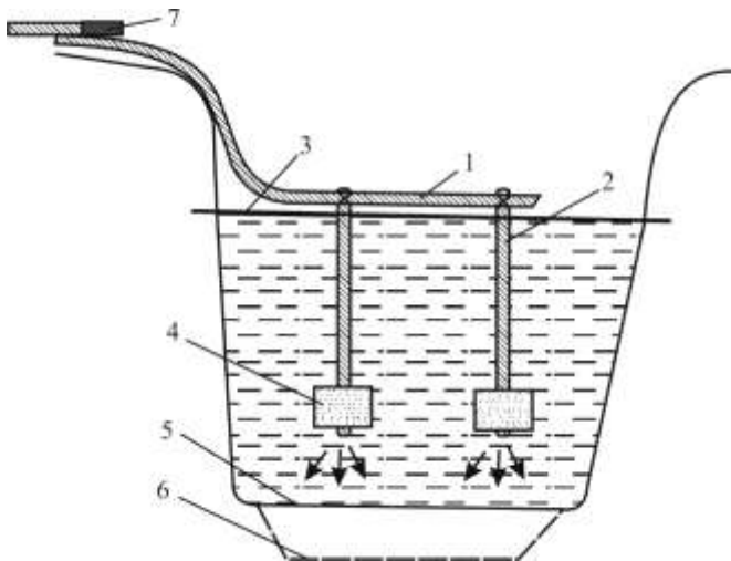
Рис. 5.2. Підвісні заряди:
