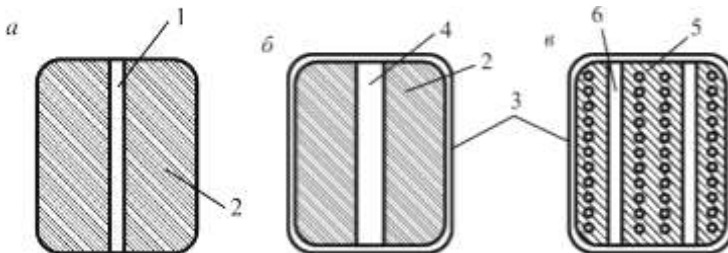
Рис. 3.13. Шашки-детонатори
