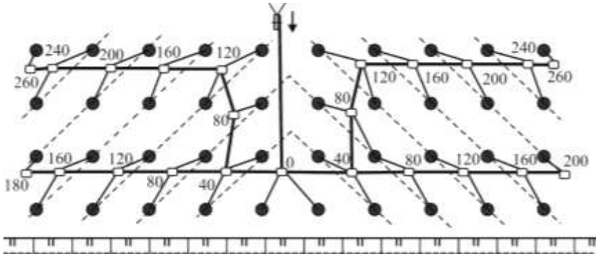
Рис. 4.36. Клинова монтажна схема ініціювання за допомогою УНС-ПА-40 або УНС-П-40
