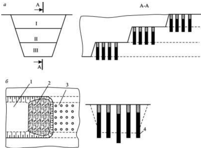
Рис. 7.25. Проходка траншей:
