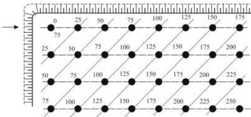
Рис. 4.32. Діагональна схема ініціювання зарядів ВР з використанням пристроїв УНС-ПА-25 або УНС-П-25
