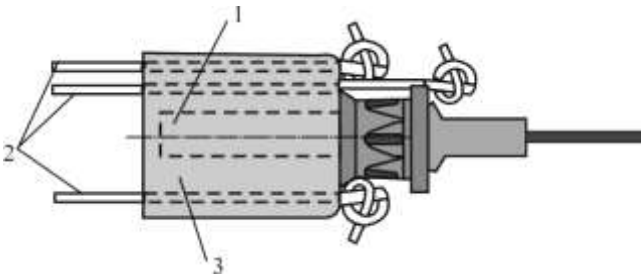
Рис. 4.27. Замок УНС-П для кріплення шести хвилеводів системи "Імпульс"
