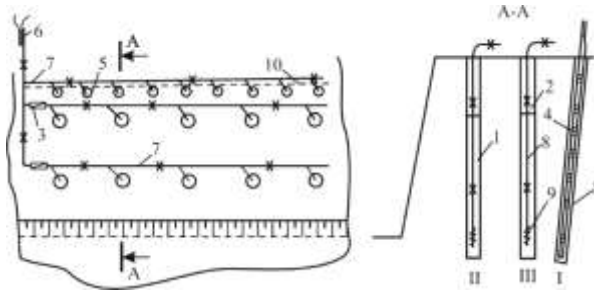
Рис. 7.20. Контурний вибух:
