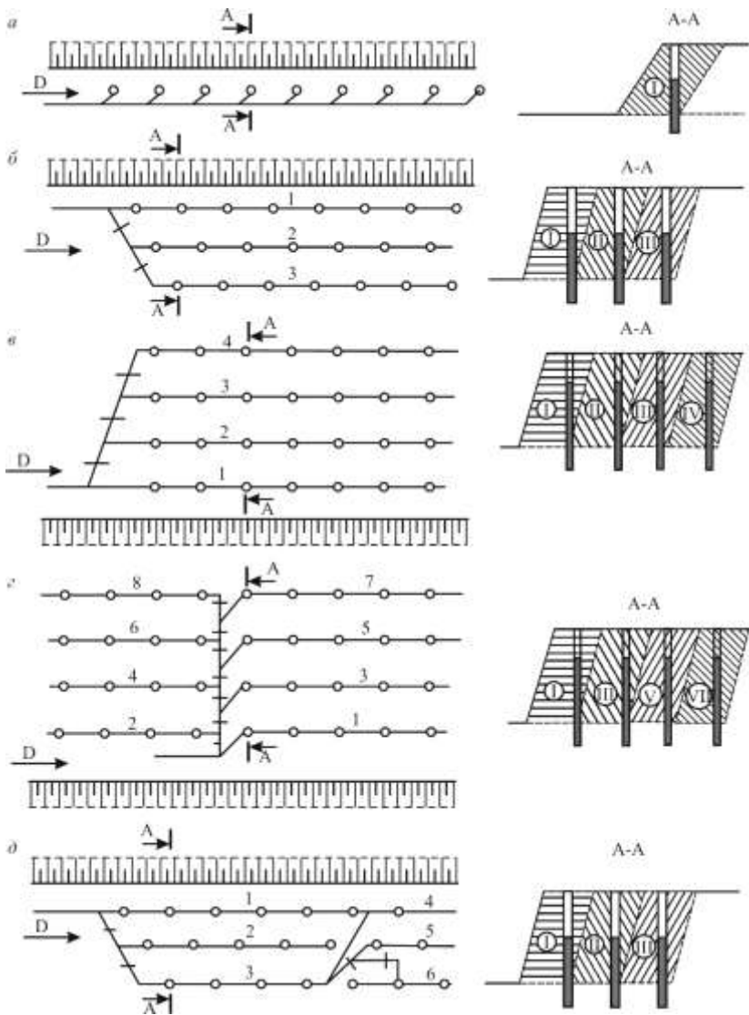
Рис. 6.8. Порядові схеми з'єднання зарядів
