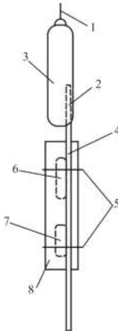
Рис. 7.10. Спеціальне пристосування, яке використовується для встановлення пристрою П-1 в обводнених свердловинах
