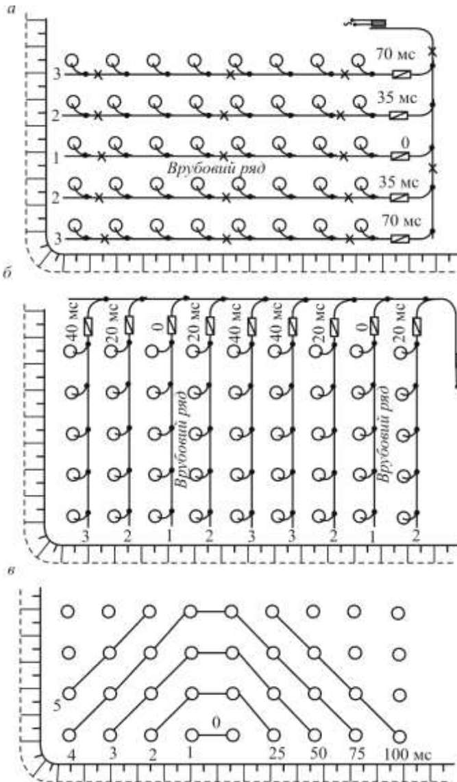
Рис. 6.7. Врубові схеми короткосповільненого багаторядного вибуху: а – з поздовжнім врубом; б – з поперечним врубом; в – з трапецеїдальним врубом; 1, 2, 3, 4, 5 – послідовність вибуху рядів зарядів
