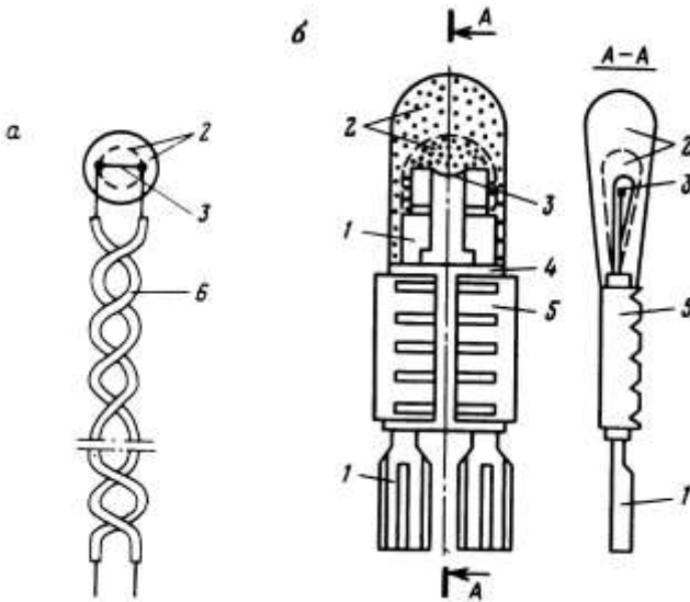
Рис. 3.6. Конструкція електрозапальників:
