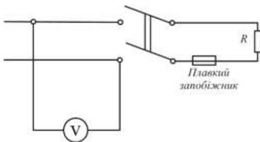
Рис. 4.2. Схема вимірювання падіння напруги в силовій мережі (джерело струму)
