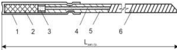
Рис. 3.3. Запалювальна трубка
