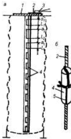
Рис. 7.22. Схема розміщення патронів ВР в шпурі
