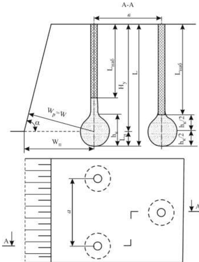
Рис. 7.11. Котлові заряди при уступному відбиванні гірської породи: H_к – висота котла; W_п – л. о. п. п
