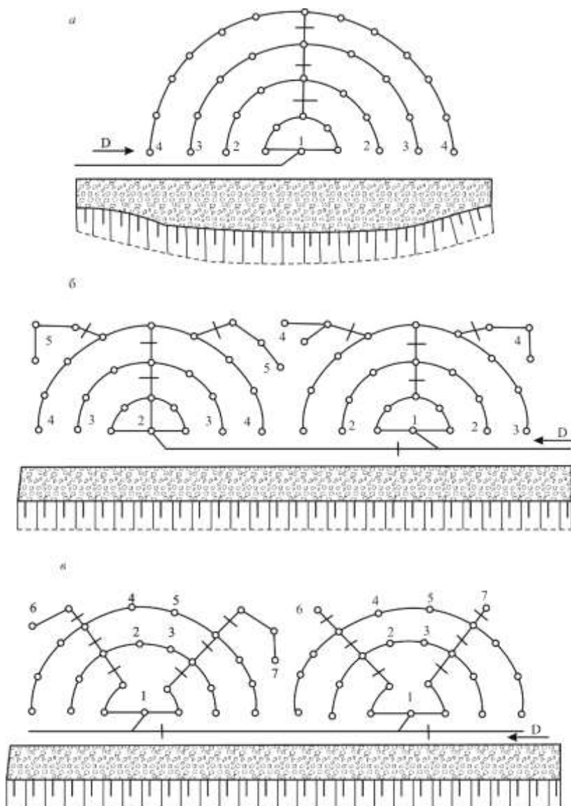
Рис. 6.14. Радіальні схеми з'єднання зарядів
