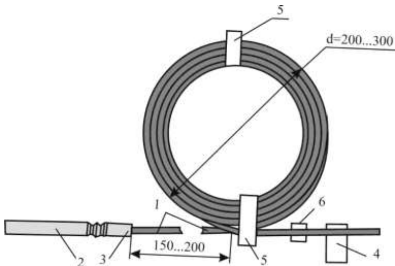
Рис. 4.25. Пристрій УНС-С
