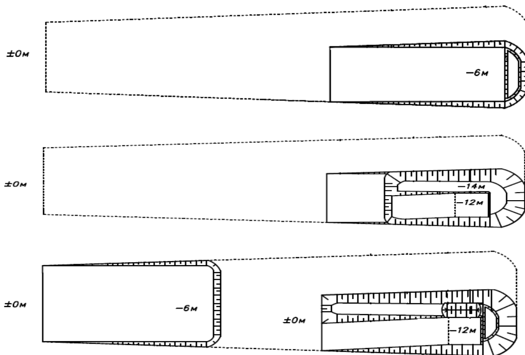
Рис. 4. Реалізація послідовної технологічної схеми ( K_{м.с} = 0,21 , K_{к.з} = 0,4 )
