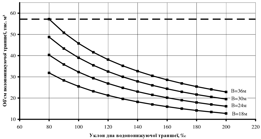
Рис. 7. Залежність обсягу водопонижувальної траншеї від уклону її дна
