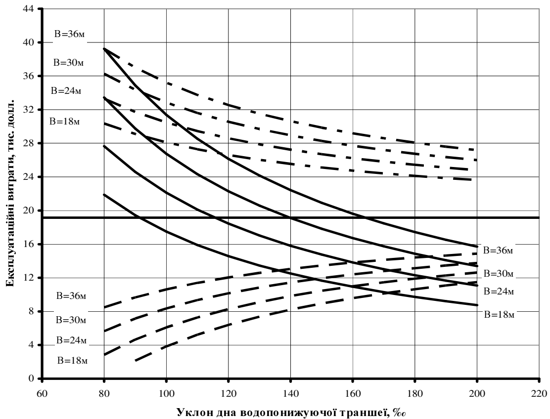
Рис. 8. Залежність експлуатаційних витрат на розкриття горизонту при послідовних технологічних схемах від параметрів водопонижувальної траншеї. Суцільними лініями позначена робота гідравлічної лопати, штриховими – механічної лопати. Штрихпунктирні лінії характеризують витрати на розкриття горизонту, окремо винесено витрати на розкриття уступу в сухих умовах (суцільна пряма)
