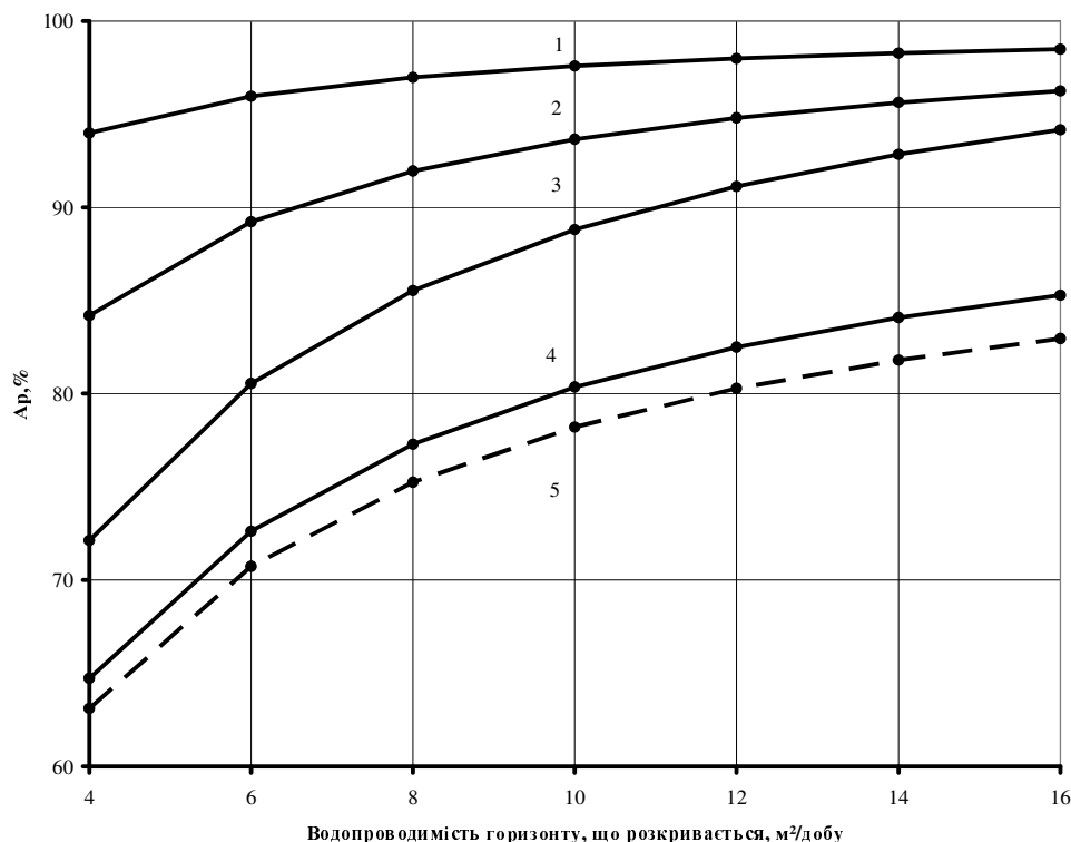
Рис. 9. Залежність відносної продуктивності кар'єру по руді від гідрогеологічних умов горизонту, що розкривається при застосуванні послідовних схем ( k_{m.c.} = 0,21 (1), k_{m.c.} = 0,45 (2)), паралельних схем ( k_{m.c.} = 0,21 (4), k_{m.c.} = 0,51 (3)) та при поширивій проходці траншеї в обводнених умовах (5)
