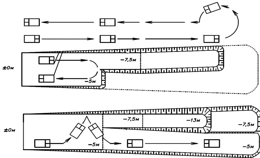
Рис. 2. Реалізація паралельної технологічної схеми ( K_{т.с.} = 0,51 , K_{к.з.} = 1 )
