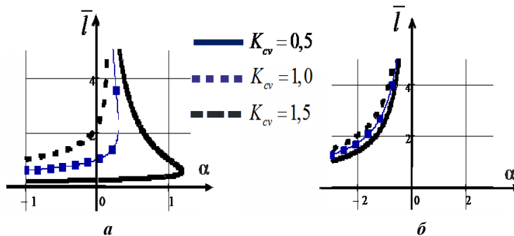
Рис. 2. Области изменения \bar{l} и \alpha , в которых возможно инициирование страгивания трещины колебательной нагрузкой при различных значениях параметра K_{cv} : а) \sigma_0 \geq 0 , б) \sigma_0 < 0
