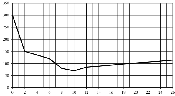
Рис. 2. Графік залежності розміру середнього куска підірваної гірської маси d від інтервалу сповільнення \tau
