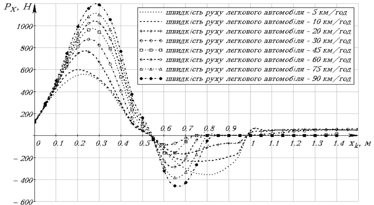
Рис. 4. Залежність поєздовжньої сили при взаємодії колеса легкового автомобіля Renault 15TS з опорною поверхнею під час його руху на різних швидкостях нерівною дорозою (параметри нерівності: синусоїдальний профіль, висота – 5 см, довжина – 1 м) від поточної координати центру колеса
