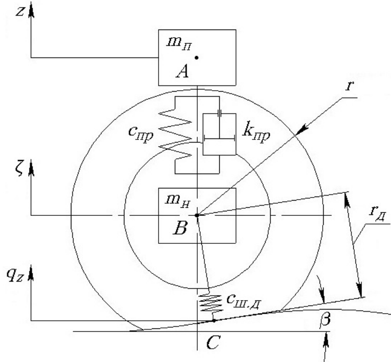
Рис.1. Розрахункова схема до визначення сил взаємодії колеса легкового автомобіля під час руху нерівною дорогою
