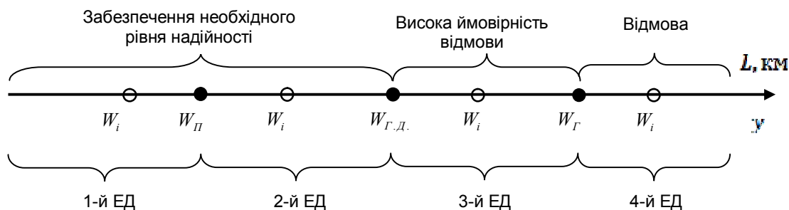
Рис. 3. Розподіл експлуатаційних діапазонів (ЕД): W_п – значення комплексного параметра, при якому виконання профілактичних робіт стає економічно доцільним; W_{г.д.} – гранично допустиме значення; W_г – граничне значення
