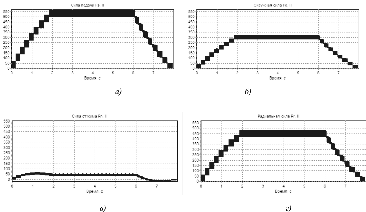
Рис. 2. Часові реалізації сил різання прорізної фрези за відсутністю радіального биття при зустрічній схемі фрезерування, Н: а – сила подачі; б – колова сила; в – сила відтиску; г – радіальна сила
