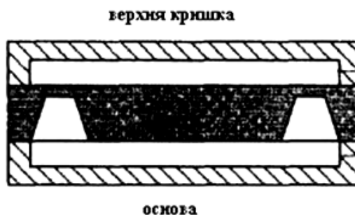
Рис. 1. Ємнісний акселерометр
