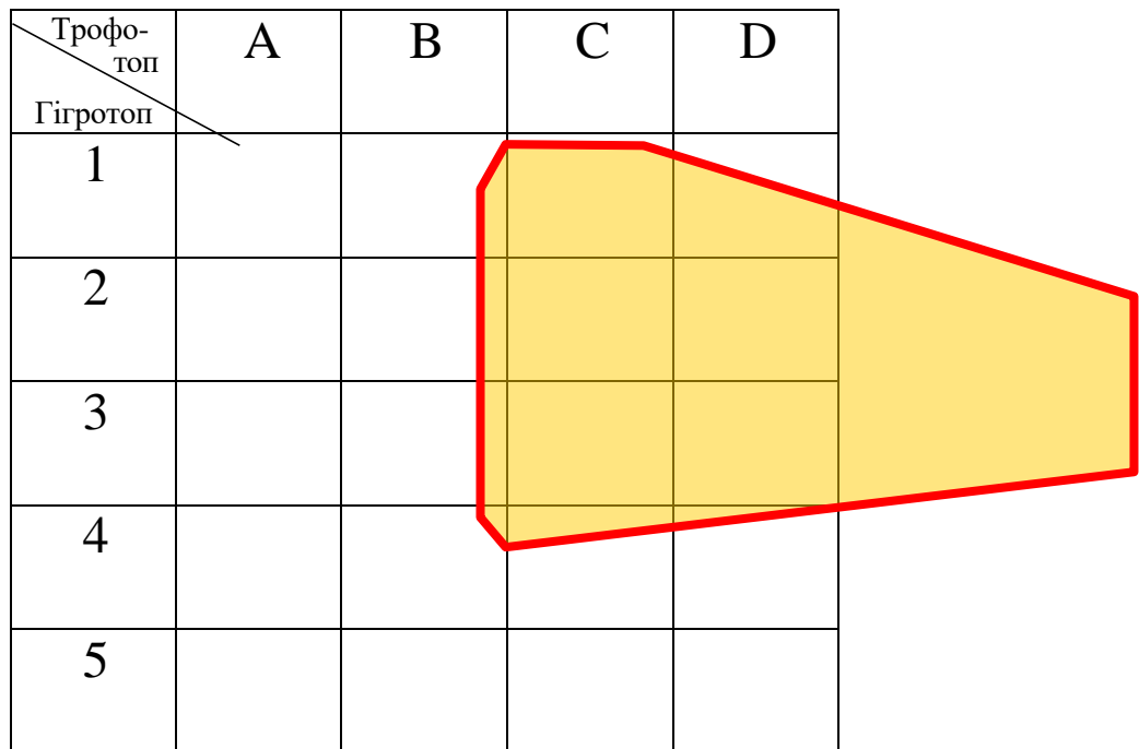
Рис. 20. Екологічний ареал лисички звичайної
