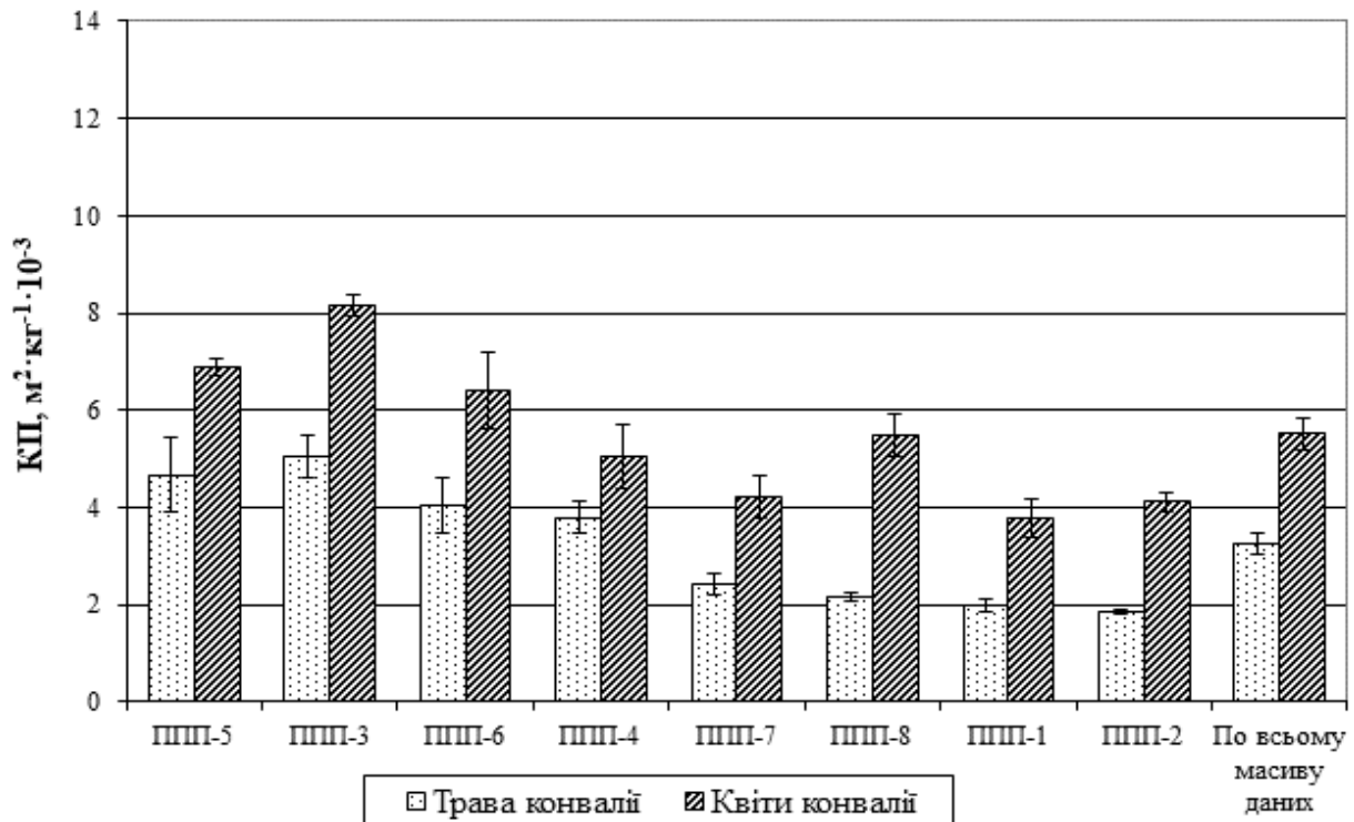
Рис. 11. Величини коефіцієнтів переходу ^{137}\text{Cs} у траву та квіти конвалії звичайної на дослідних ділянках у 2018 р. ( \text{м}^2 \cdot \text{кг}^{-1} \cdot 10^{-3} )
