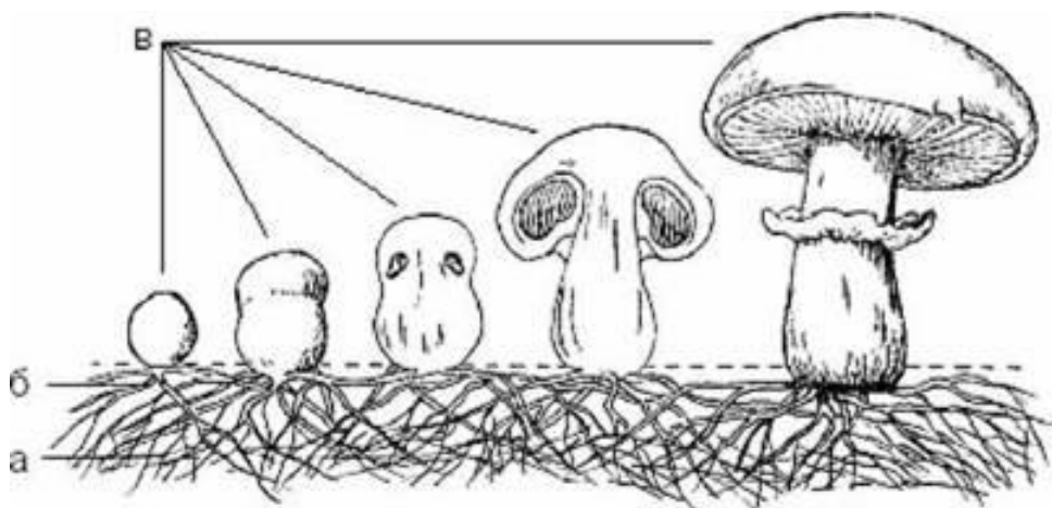
Рис. 16. Міцелій і плодові тіла грибів: а – гіфи; б – міцелій; в – плодові тіла
