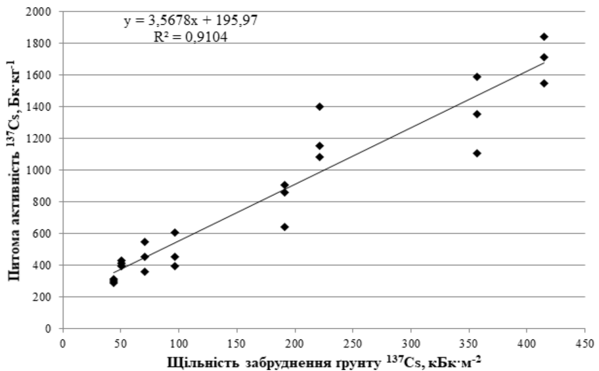
Рис. 12. Залежність питомої активності ^{137}\text{Cs} у траві (а) і суцвіттях (б) конвалії звичайної від щільності забруднення ґрунту радіонуклідом у 2018 р
