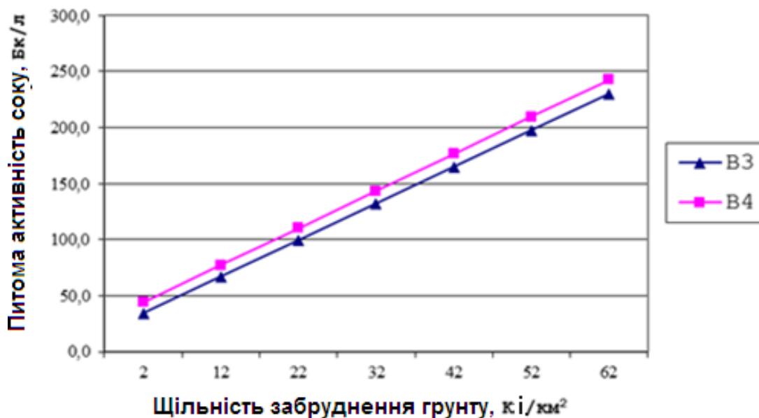
Рис. 27. Залежність питомої активності 137 Cs у березовому соку від щільності радіоактивного забруднення ґрунту в різних умовах місцезростання
