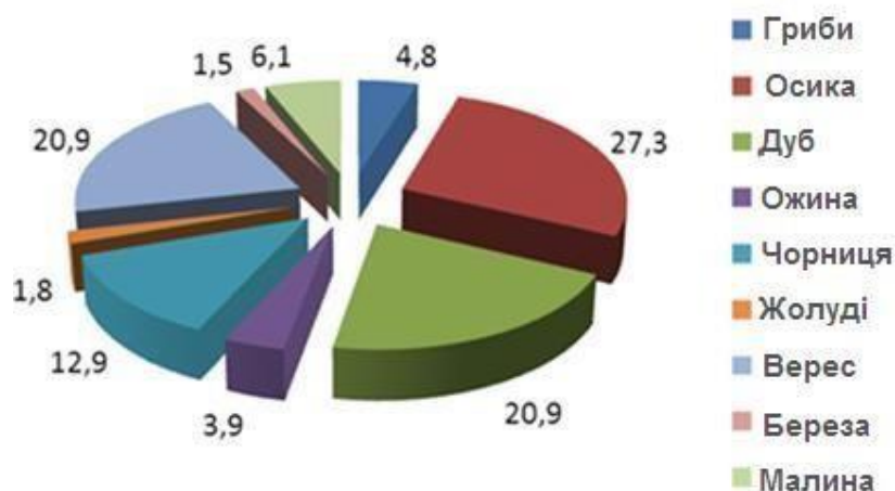
Рис. 34. Структура радіоактивного забруднення осіннього раціону косулі європейської на Поліссі України, % від сумарної активності ^{137}\text{Cs} у раціоні
