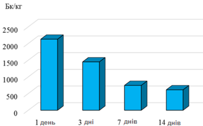
Рис. 35. Зміна питомої активності 137 Cs в ягодах брусниці при замочуванні
