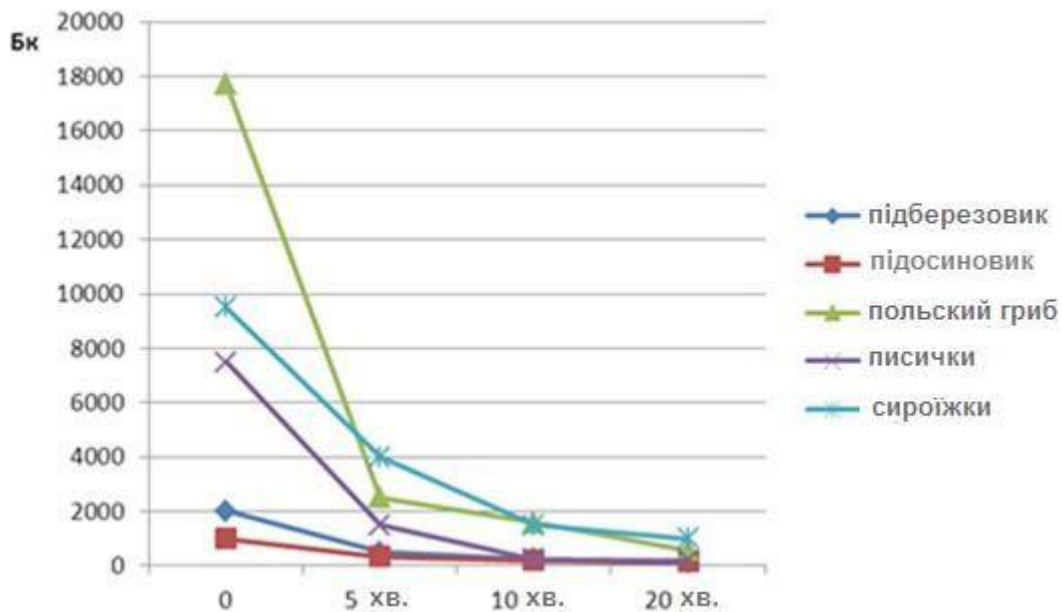
Рис. 37. Зміна вмісту ^{137}\text{Cs} у свіжих плодових тілах грибів у процесі відварювання
