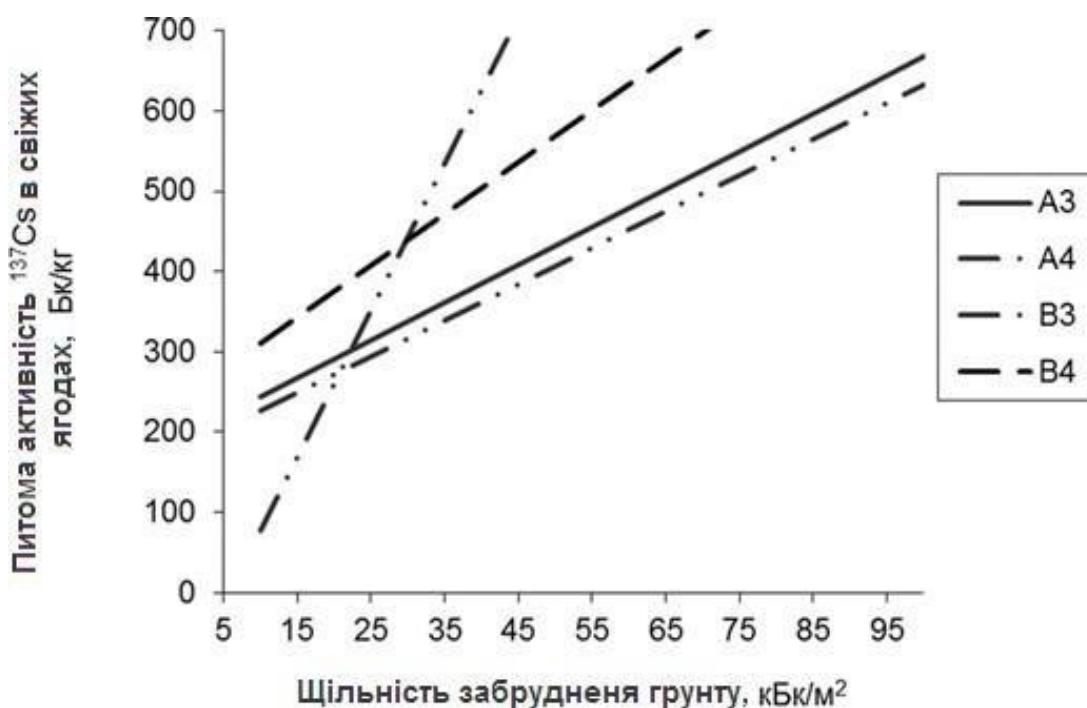
Рис. 6. Питома активність ^{137}\text{Cs} у свіжих ягодах брусниці при різній щільності забруднення ґрунту в основних типах умов місцезростання
