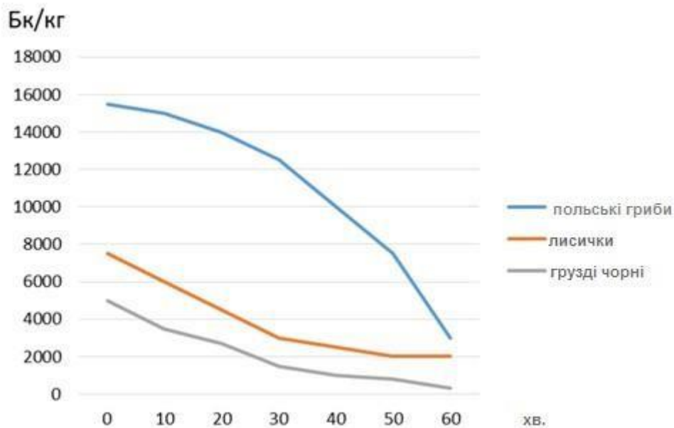
Рис. 38. Зміна сумарної активності ^{137}\text{Cs} у плодівих тілах їстівних грибів у процесі їх вимочування
