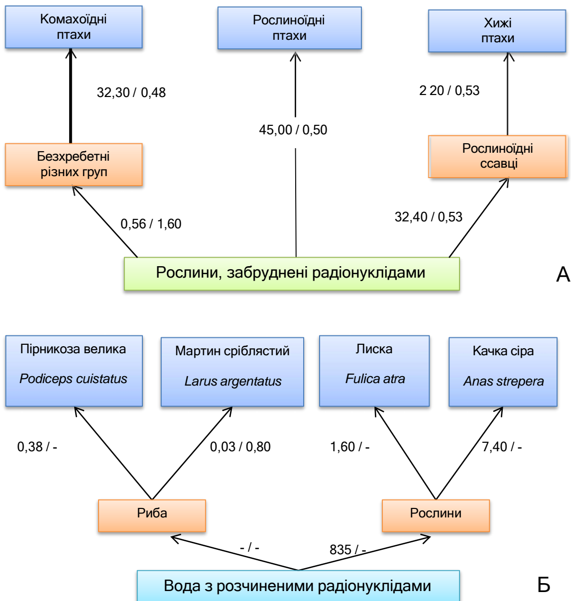
Рис. 29. Середні значення коефіцієнтів концентрації ^{90}\text{Sr} (над рискою) і ^{137}\text{Cs} (під рискою) для різних груп птахів в наземному (А) і прісноводному (Б) зооценозах
