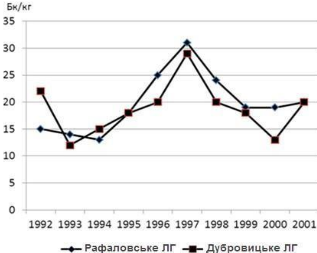
Рис. 25. Особливості радіоактивного забруднення березового соку протягом 10 років (1992–2001 рр.)
