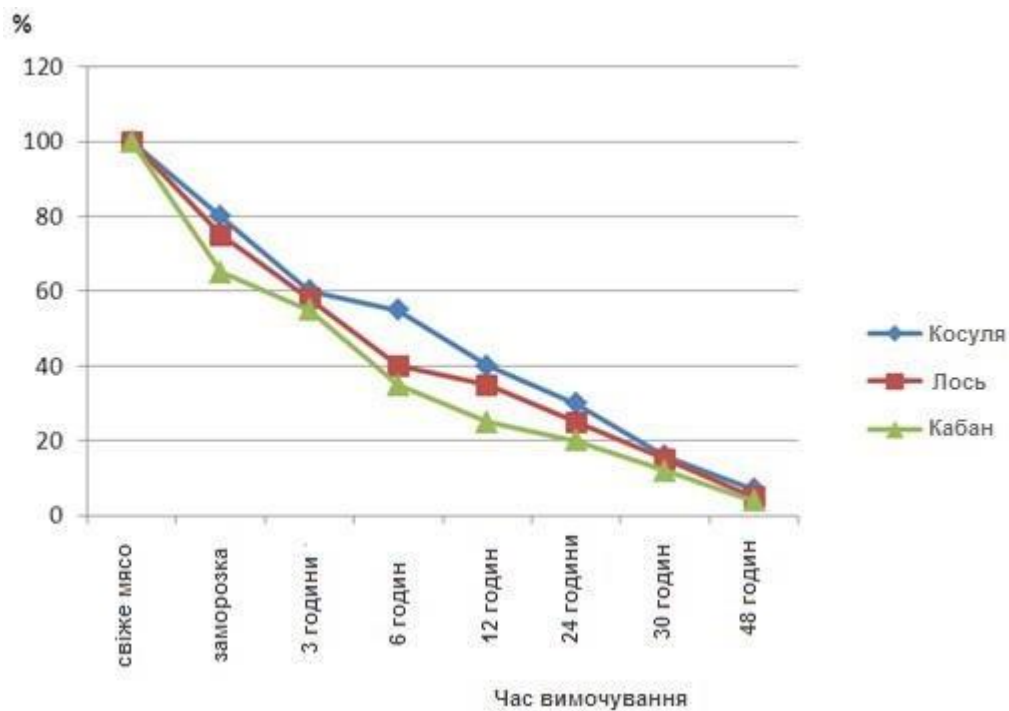
Рис. 39. Відносна зміна питомої активності ^{137}\text{Cs} у м'ясі мисливської дичини в процесі вимочування
