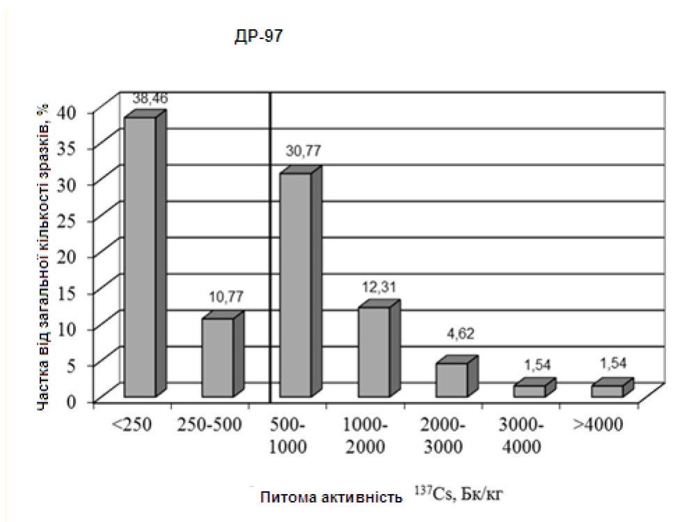
Рис. 17. Розподіл зразків свіжих плодових тіл грибів за діапазонами питомої активності 137 Cs (згідно із даними радіологічного контролю в Житомирській області за 2002–2004 рр.)
