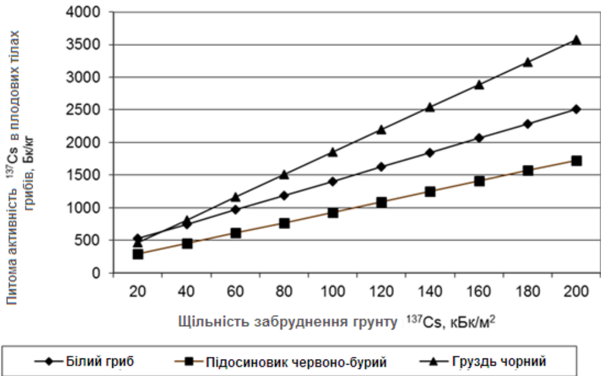
Рис. 18. Номограми для визначення вмісту ^{137}\text{Cs} у плодкових тілах грибів при різній щільності радіоактивного забруднення ґрунту
