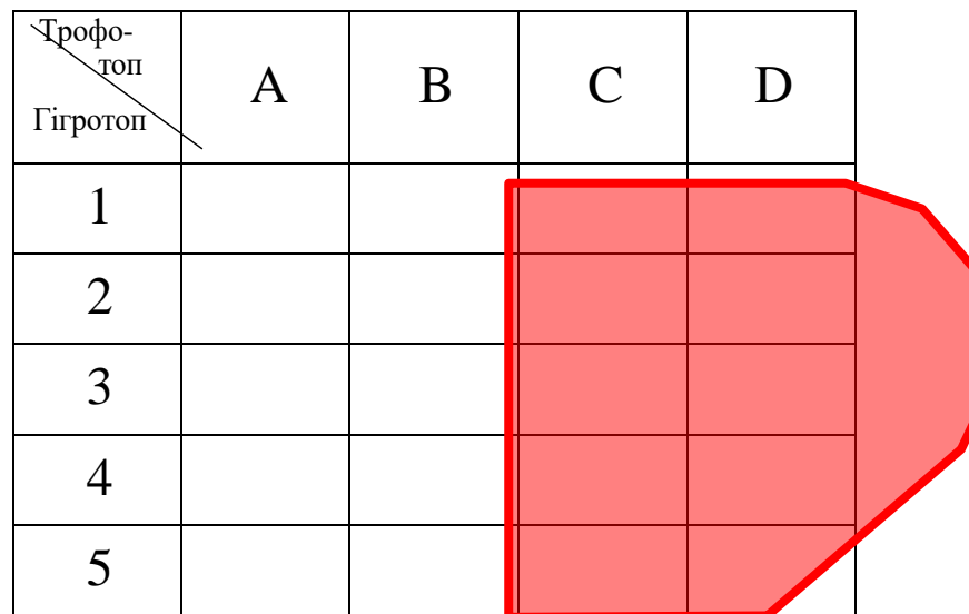
Рис. 23. Екологічний ареал моховика тріщинуватого
