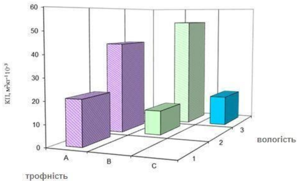
Рис. 21. Коефіцієнт переходу 137 Cs у плоді тіла лисички в різних типах лісорослинних умов
