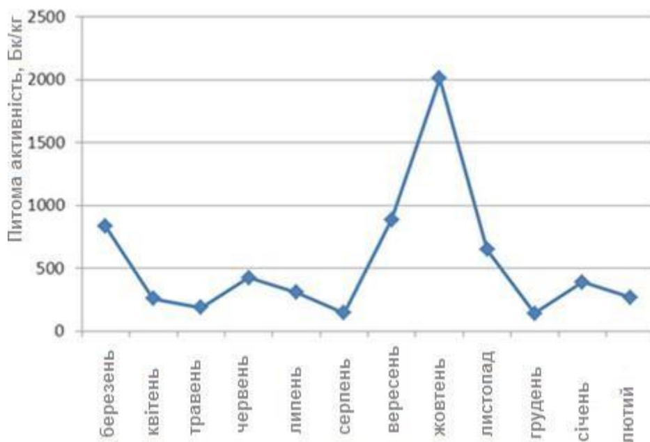
Рис. 33. Сезонна динаміка накопичення ^{137}\text{Cs} у м'язах косулі європейської на Поліссі України
