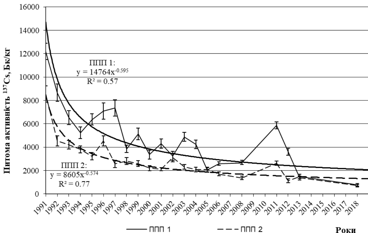
Рис. 13. Динаміка питомої активності ^{137}\text{Cs} у траві конвалії на ППП-1 і ППП-2 протягом 1991-2018 р.р
