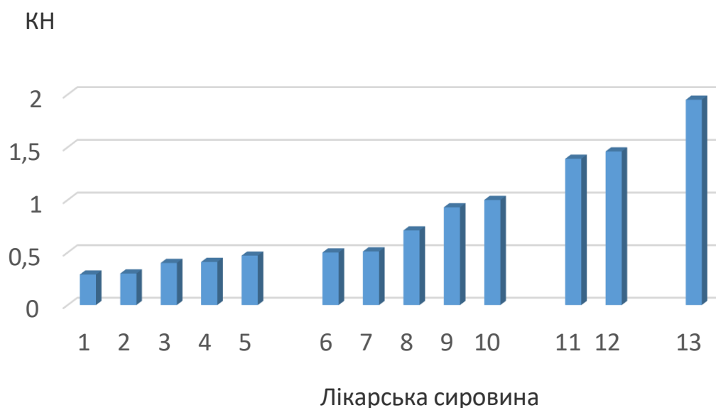
Рис.10. Групи лікарський рослин (сировини) за середніми значеннями КН ^{137}\text{Cs} у свіжих суборах
