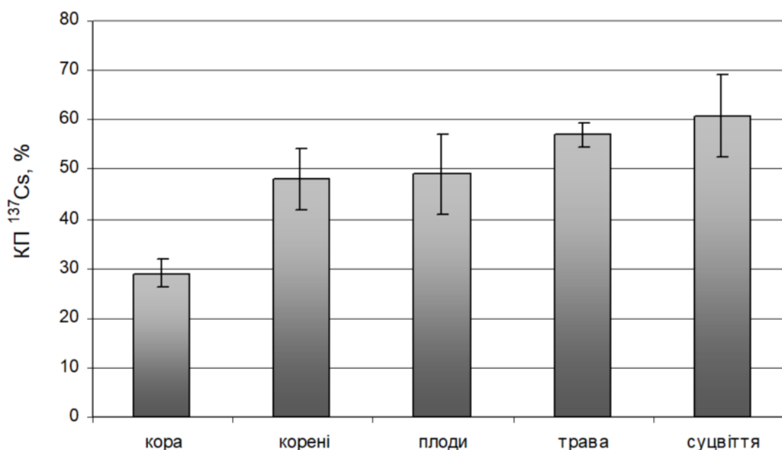
Рис. 15. Середні значення КП ^{137}\text{Cs} до лікарських форм із різних груп лікарської сировини
