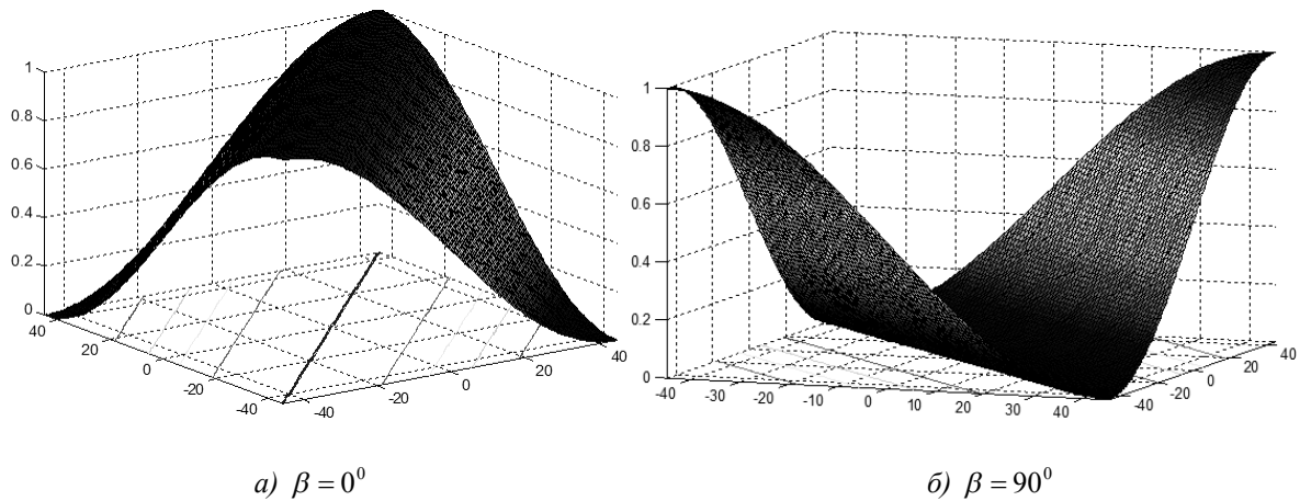
Рис. 2. Двовимірні функції поляризаційного прийому (вісь \alpha_a – ліво; вісь \alpha_c – право)
