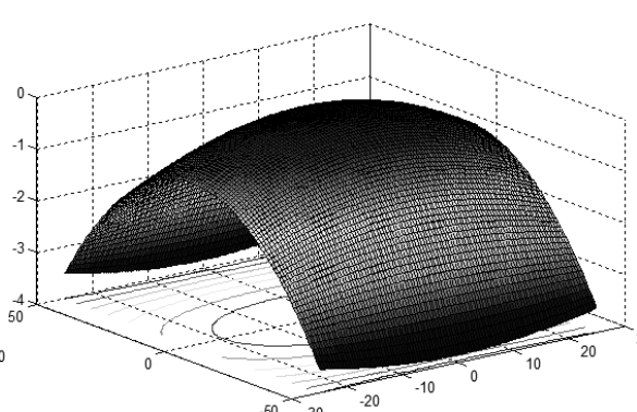
Рис. 4. Відносний поляризаційний коефіцієнт прийому \gamma_r антени лінійної поляризації (вісь \beta_c – ліво; вісь \alpha_c – право)
