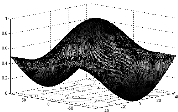
Рис. 3. Поляризаційний коефіцієнт прийому антени лінійної поляризації (вісь \beta_c – ліво; вісь \alpha_c – право)
