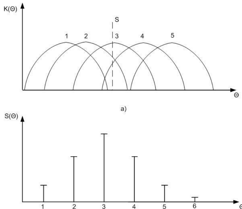
Рис.1. Формування сигнальної групи на виході ЦАР з БПДС
